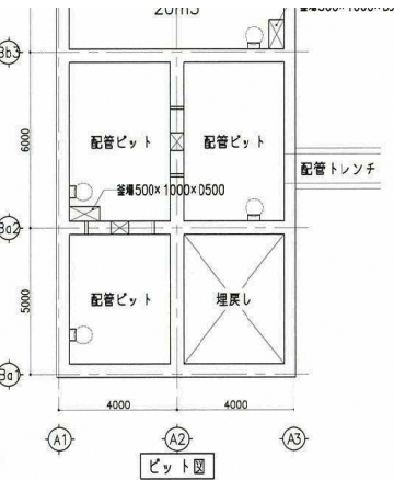
ピット図
