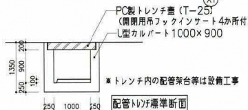
配管トレンチ標準断面
