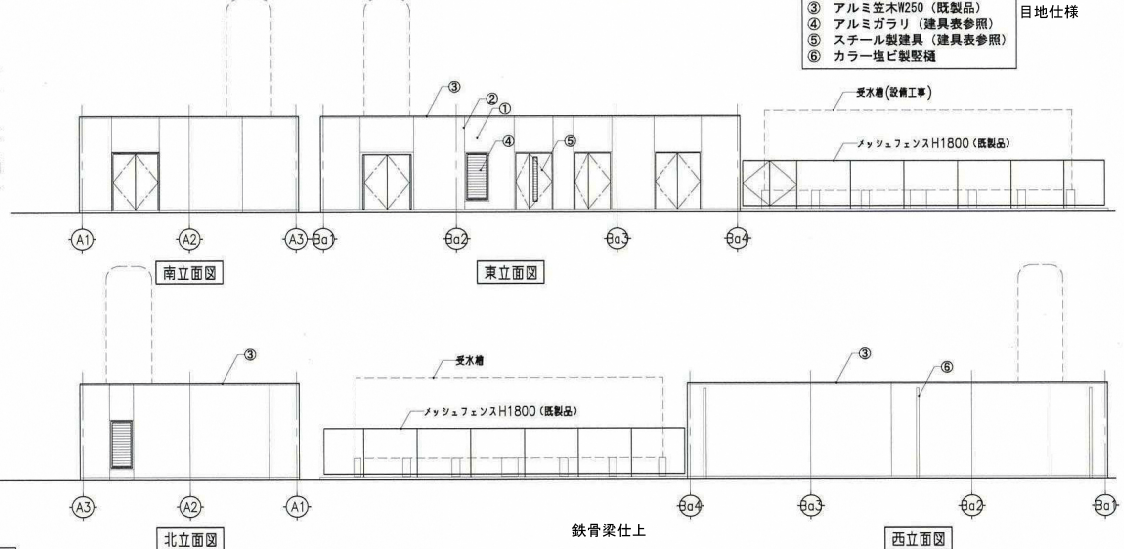
北立面図
