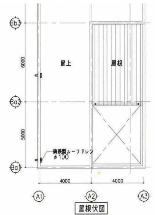
屋根伏図
